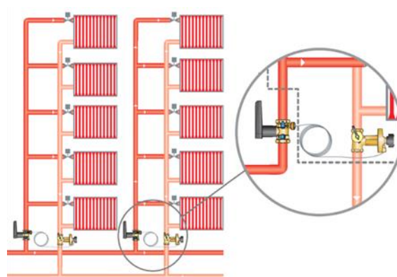
Рис. 14 Ballorex Vario установлен вне регулируемого контура
