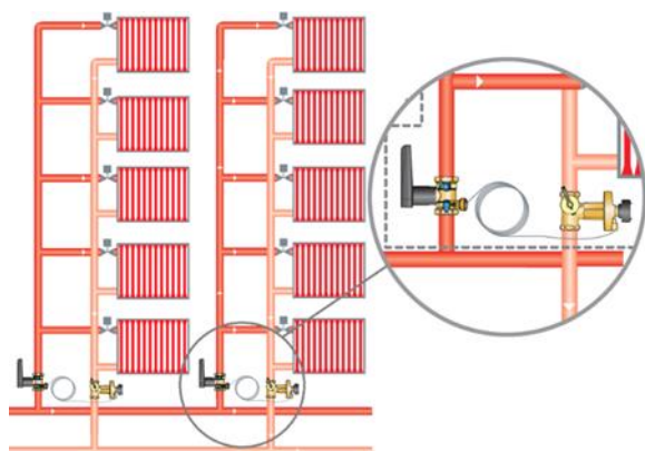
Рис. 13 Ballorex Vario установлен внутри регулируемого контура
