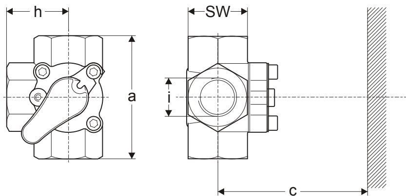
Рис. 1. Размеры V5433A
