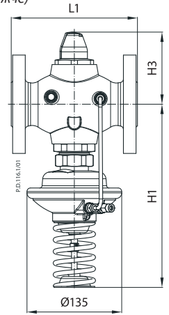
AVPQ DN 32-50 \Delta p_s = 0,3-2,0 бар
