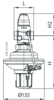
AVPQ DN 15-50 \Delta p_s = 0,2-1,0 бар
