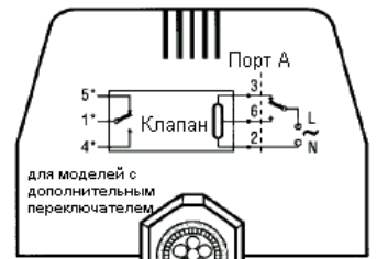
для моделей с дополнительным переключателем с витым проводом
